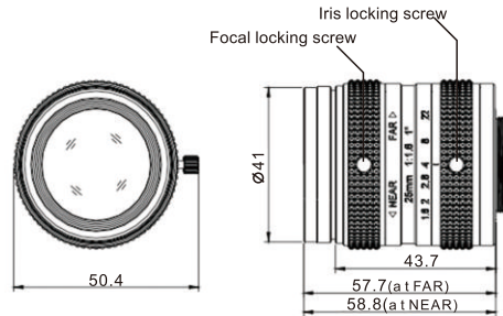
Unit : mm
